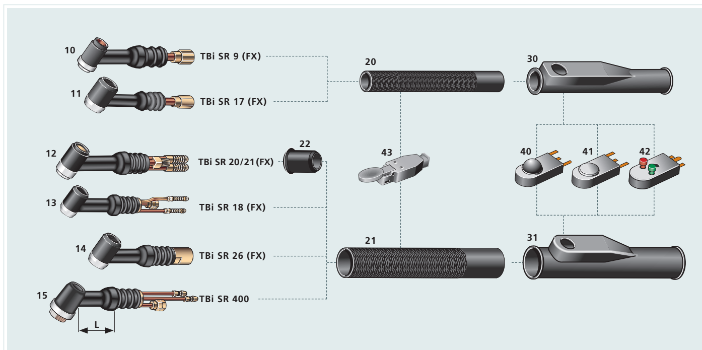
Griffrohre und Schalter / Handle tubes and switches / Poignées tubulaires et gâchettes
