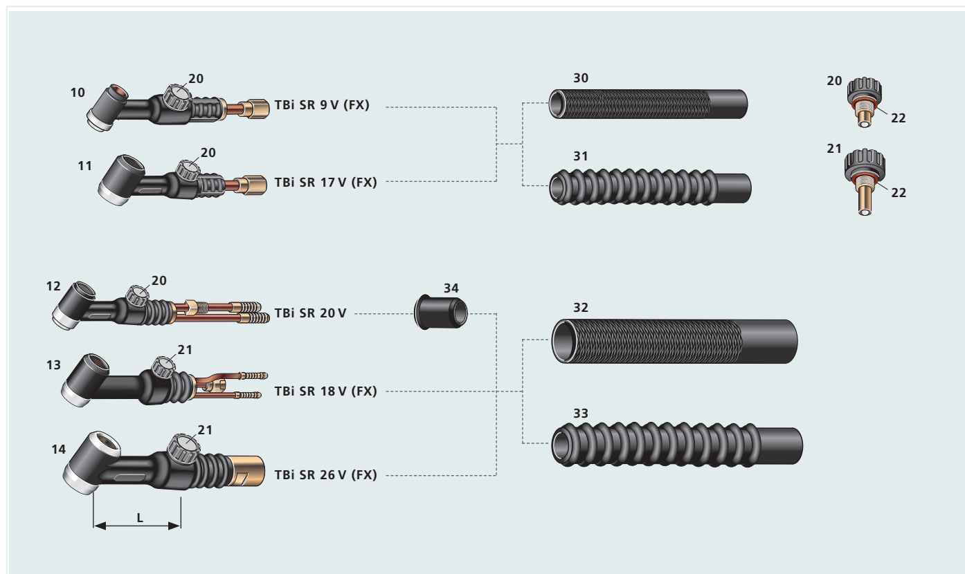
Griffrohre für Ventilbrenner / Handle tubes for torch bodies with valve / Poignées pour version à valve
